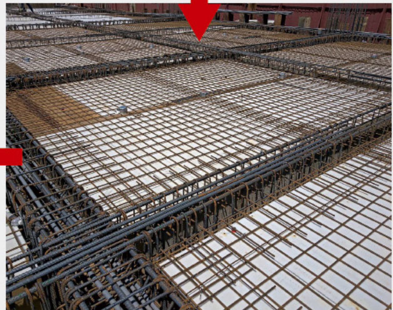
樓版鋼網下層鋪設
